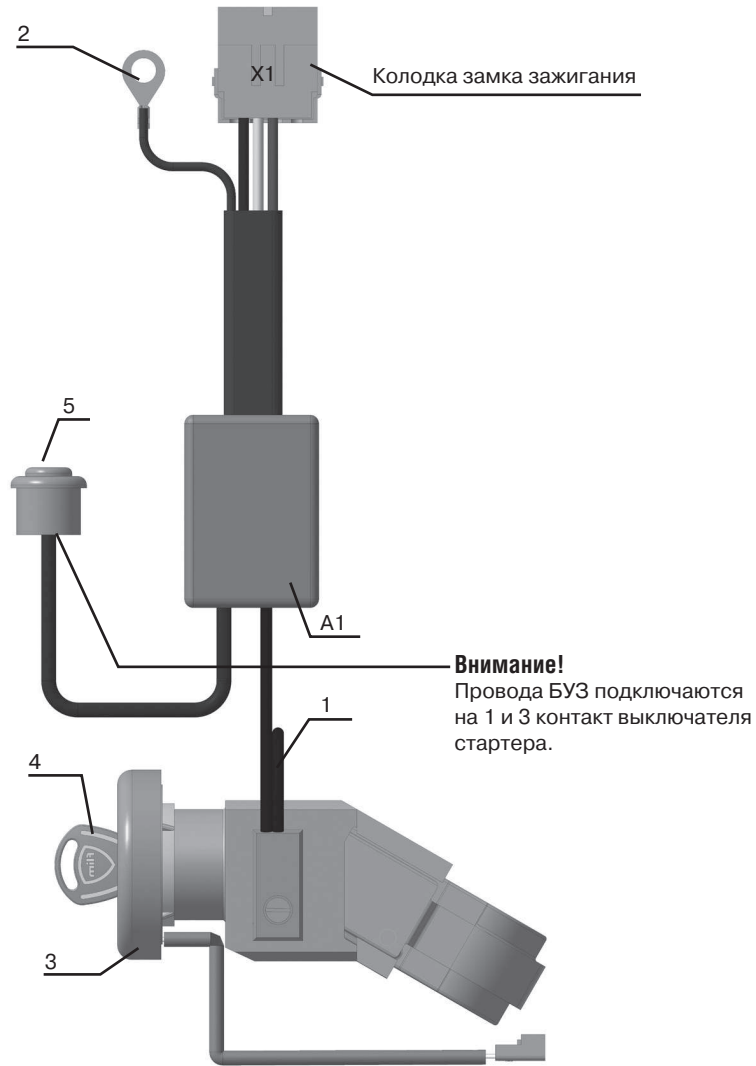
Рис. 6 Порядок подключения блока управления зажига- нием замка «Гарант Басти- он серии SINGLE»
